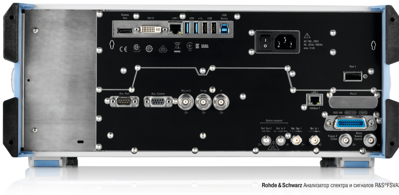
Вид задней панели прибора R&S®FSA3000
